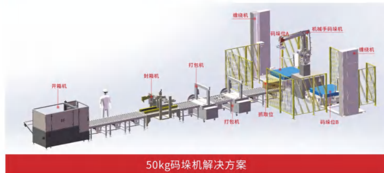
立柱码垛机解决方案
