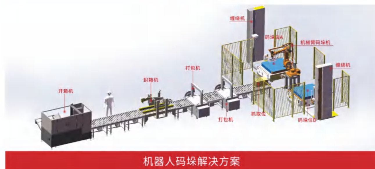
50kg码垛机解决方案
